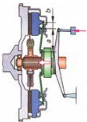
شکل ۱۸- کلاچ در حال آزاد شدن
